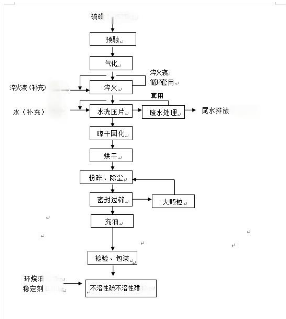
图 2.5-1 不溶性硫磺生产工艺流程图
