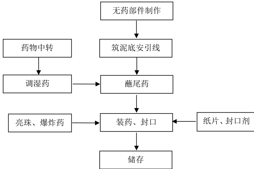
图 2.4-2 效果内筒生产工艺流程图
