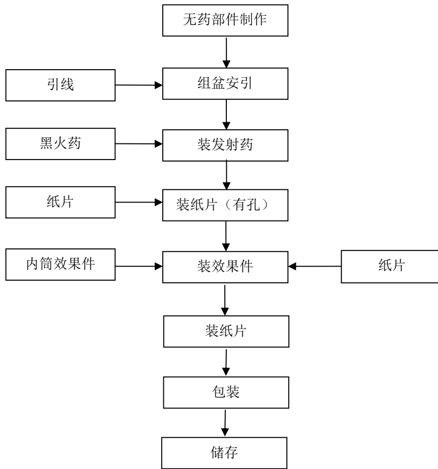
图 2.4-3 组合烟花生产工艺流程图(内筒型)
