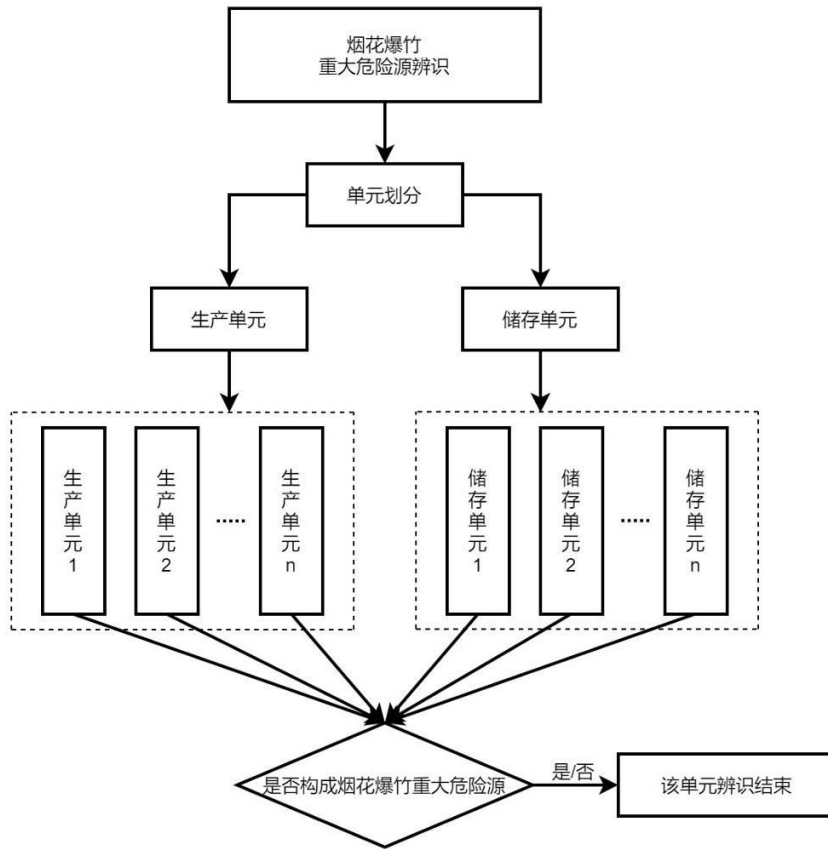
图 3.6-1 烟花爆竹重大危险源辨识流程图
