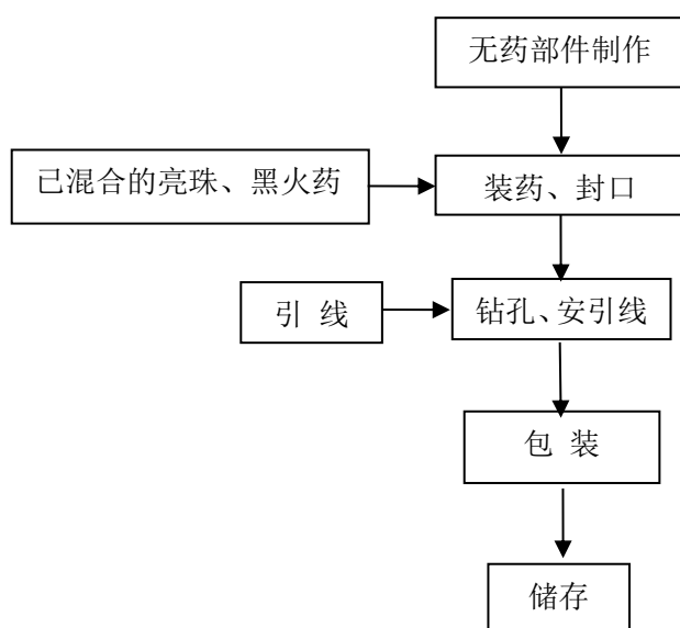
图 2.3-6 喷花类产品生产工艺流程图
