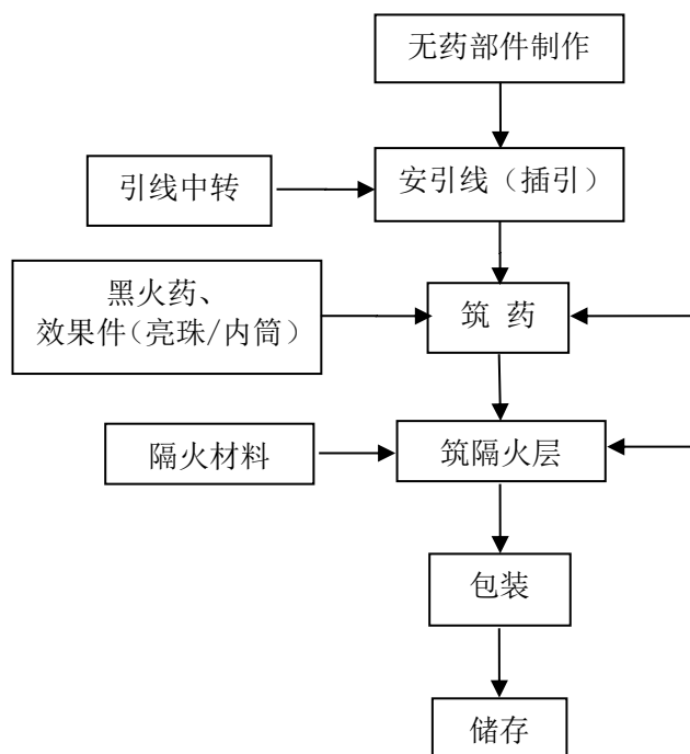
图 2.3-6 喷花类产品生产工艺流程图
