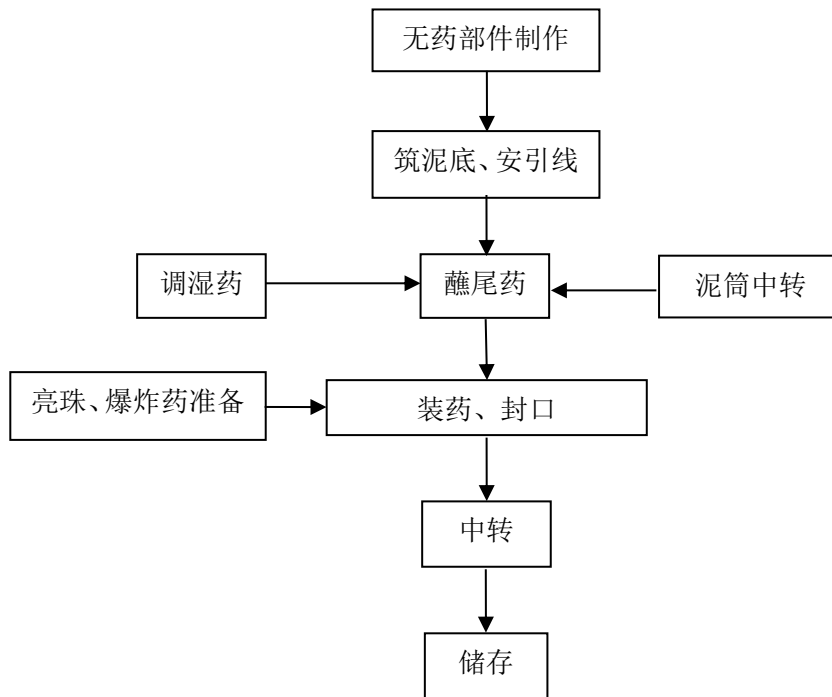
图 2.3-3 效果件内筒（机械装内筒）生产工艺流程图
