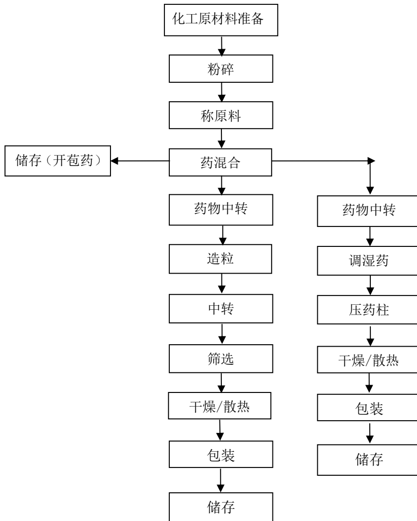
图 2.3-1 药物裸药效果件（亮珠、药柱、开苞药）生产工艺流程图
