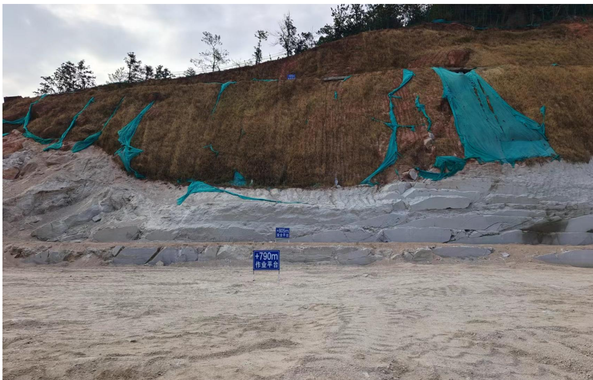
+820m、+805m 安全平台和+790m 作业平台
